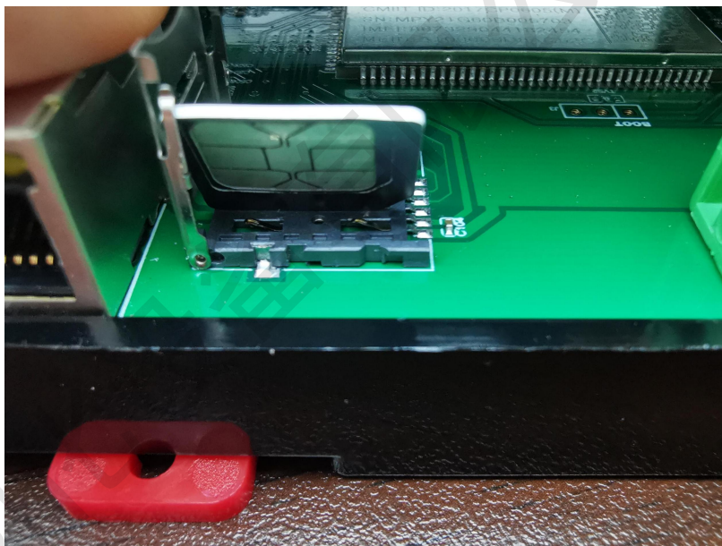
图4-1 安装SIM卡-C型
